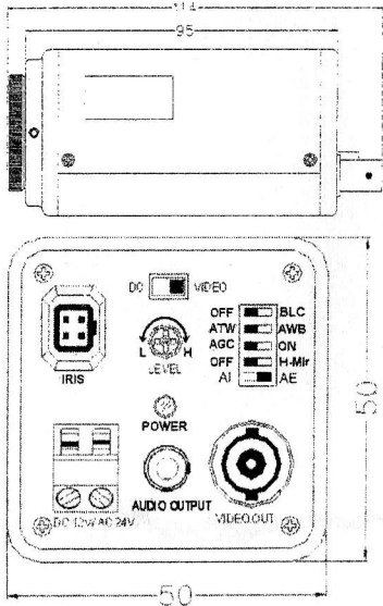
DIMENSION (UNIT:mm)
